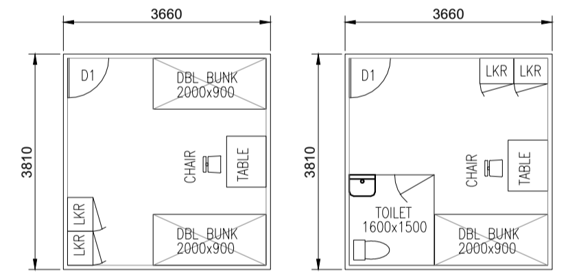
4MEN ROOM DET. 2MEN ROOM DET.
